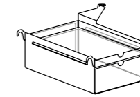
Ablagefach links: #39263 rechts: #39264 B/H/T: 24/14/35 cm · für alle RackPod-Modelle · Blech, schwarz gepulvert · 2 x Acrylauszüge: B/H/T: 23/3/35 und 23/9/35 cm
