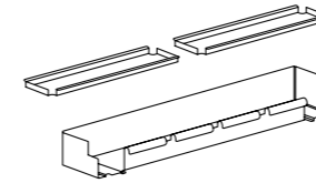
Multibox #39262 B/H/T: 79/12/12 cm · für RackPod S und H · Blech, schwarz gepulvert · zwei, mit Kork gepolsterte Ablageschalen
