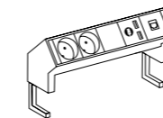
Technikanschluss ON weiß: #58283 schwarz: #58284 · für alle RackPod-Modelle · 2x Schuko, 1x USB doppelt, 1x RJ45 · mit Zuleitung und Befestigung · Gehäuse und Haltewinkel aus Aluminium
