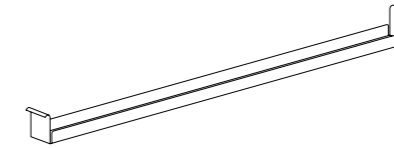
Kabelwanne S #38936 B/H/T: 150/10/12 cm · für RackPod S und H · Blech, schwarz gepulvert
